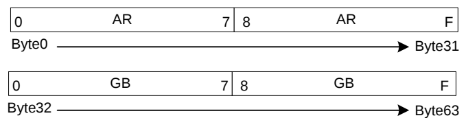
32bit Format : 4x4 texels / 2 cache lines
